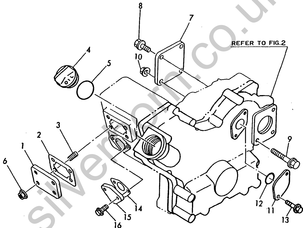
Fig. 3 ギヤケースメクラフタ GEAR HOUSING BLIND COVER
