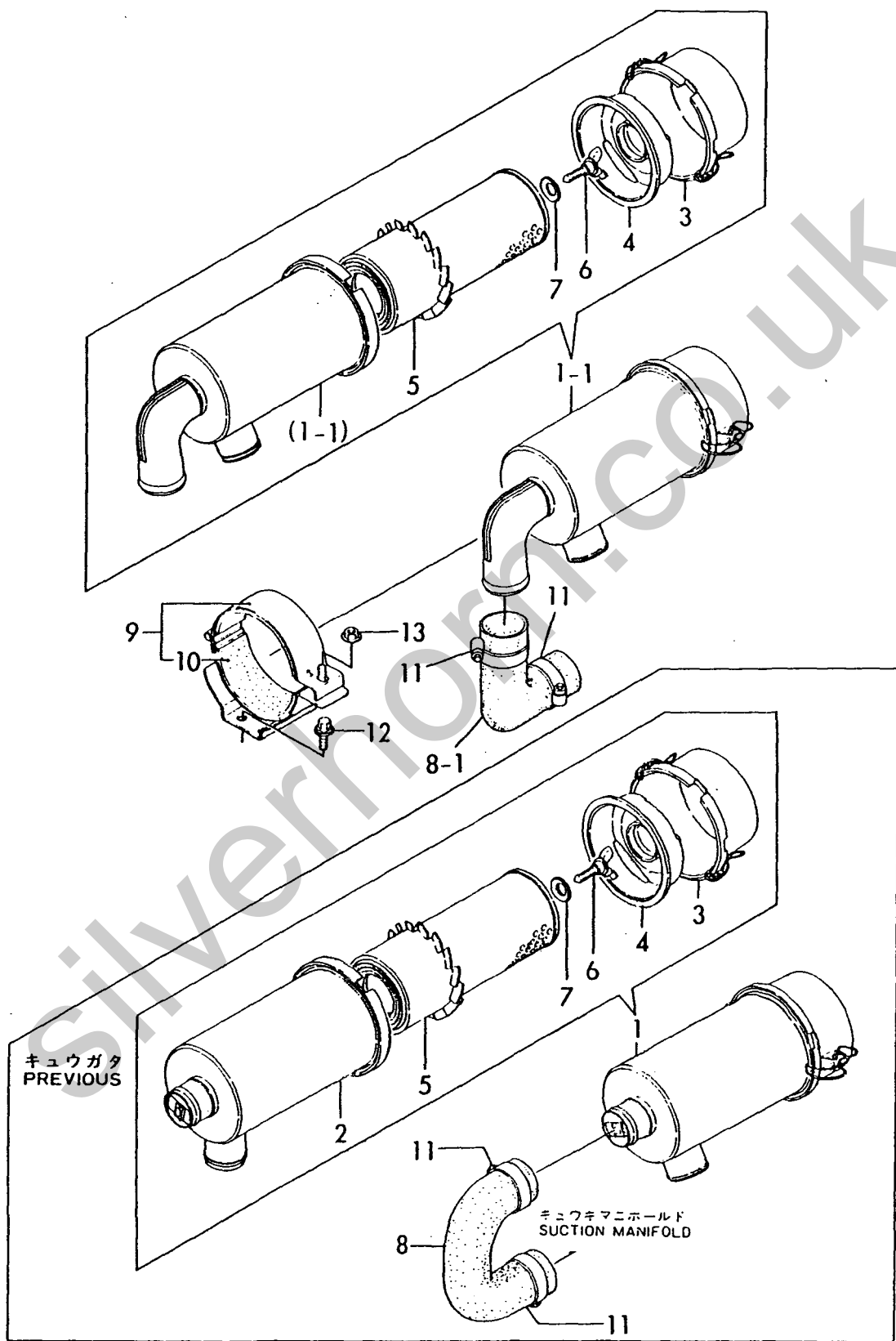
Fig. 10 エアクリーナ AIR CLEANER
