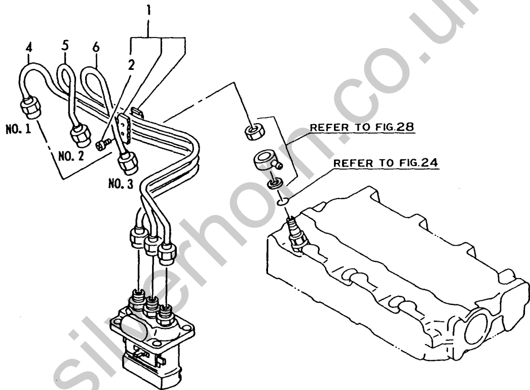
Fig. 26 FOフンシャパイプ FUEL INJECTION LINE
