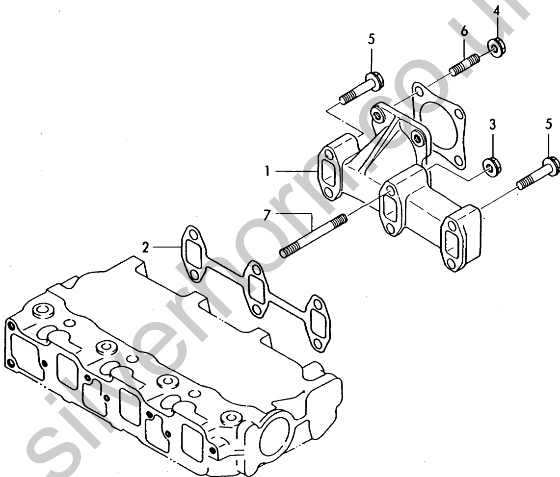
Fig. 12 ハイキマニホールド EXHAUST MANIFOLD
