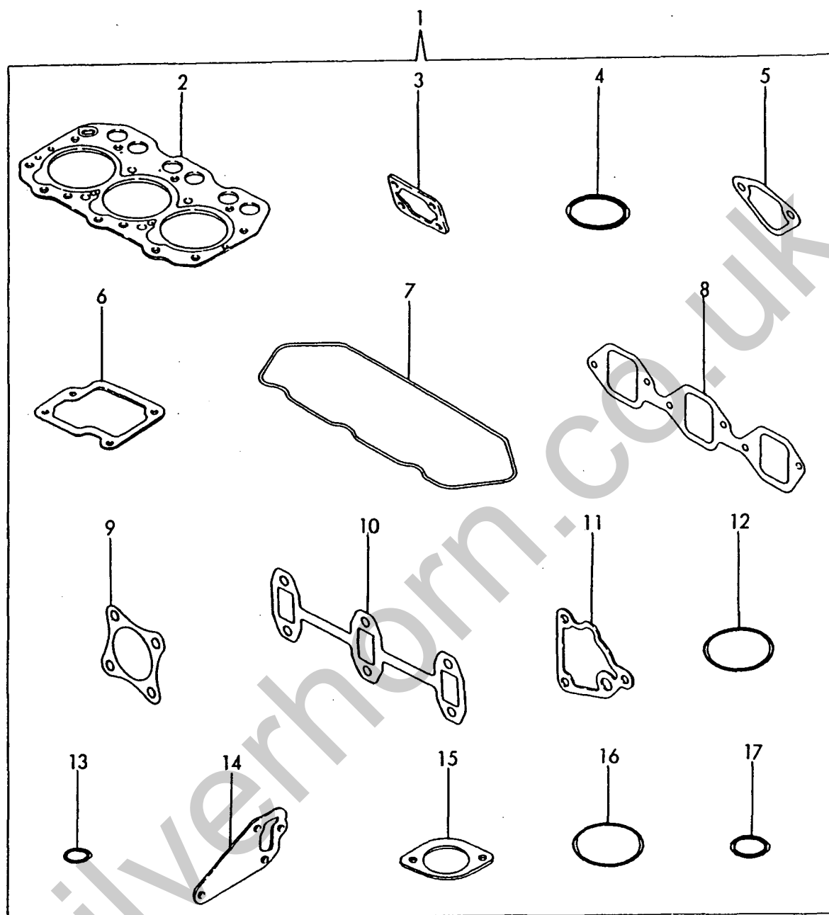
Fig. 34 パッキンセット & トクシュコウグ(オプション) GASKET SET & SPECIAL TOOL (OPTIONAL)
