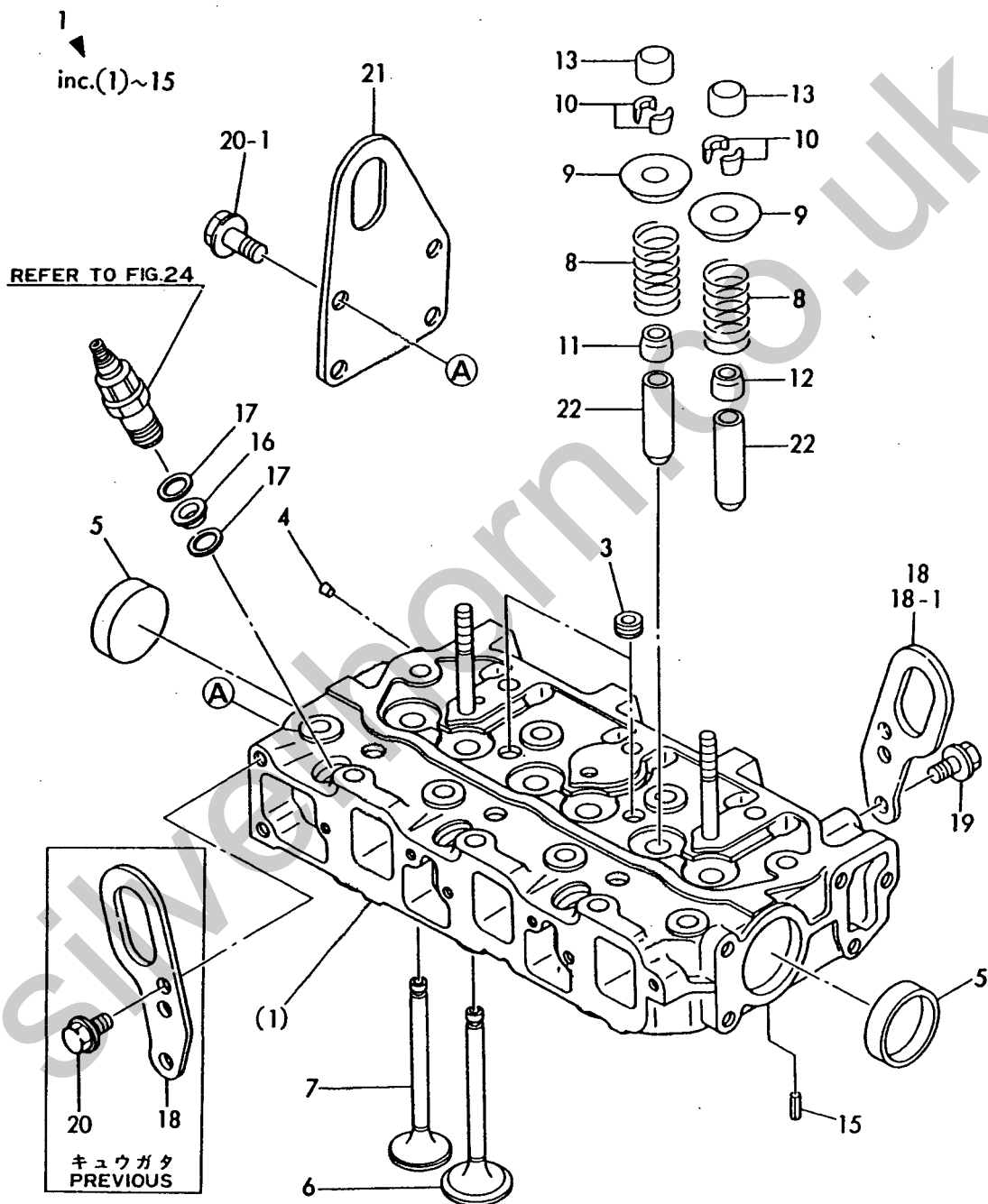
Fig. 7 シリンダヘッド CYLINDER HEAD
