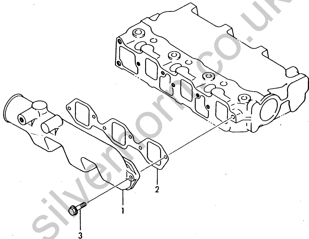
Fig. 11 キュウキマニホールド SUCTION MANIFOLD
