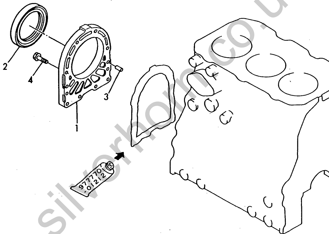
Fig. 5 オイルシールケース OIL SEAL HOUSING
