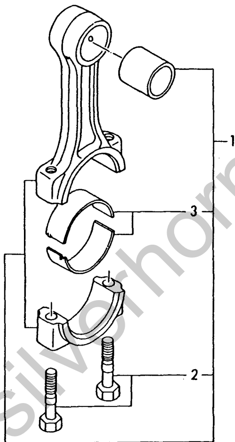
Fig. 17 コネクティングロッド CONNECTING ROD
