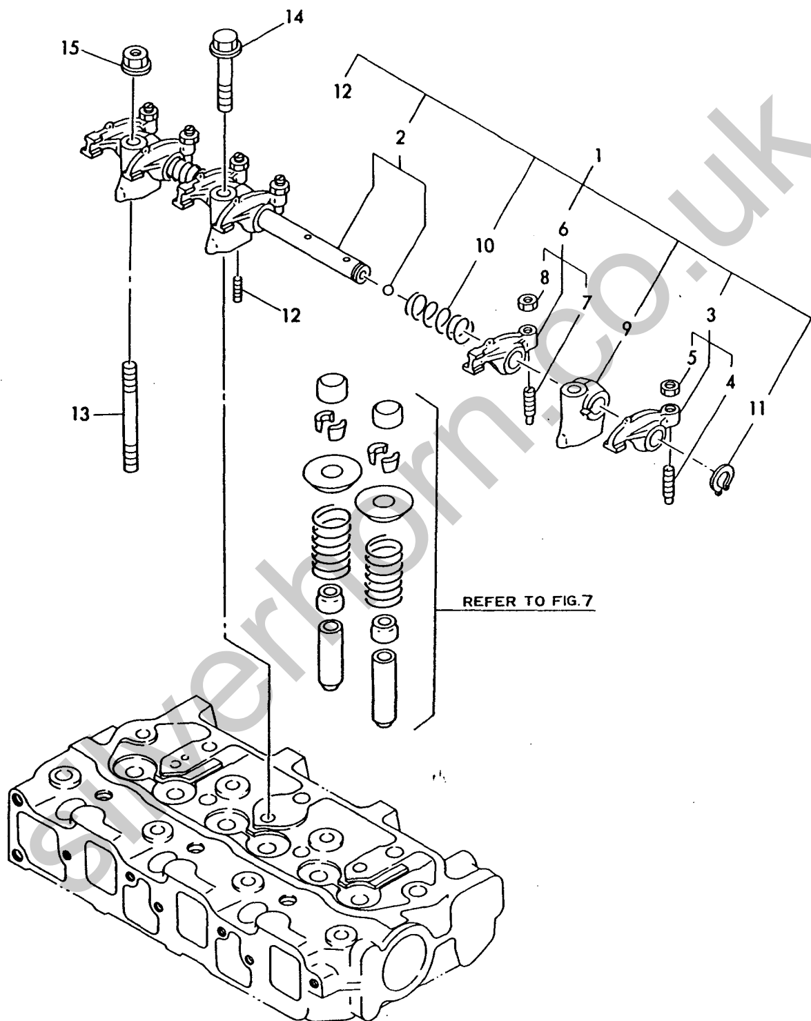
Fig. 8 ペンワン ROCKER ARM
