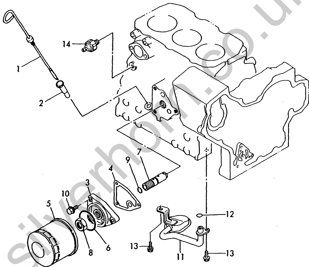
Fig. 20 LOシステム LUB. OIL SYSTEM
