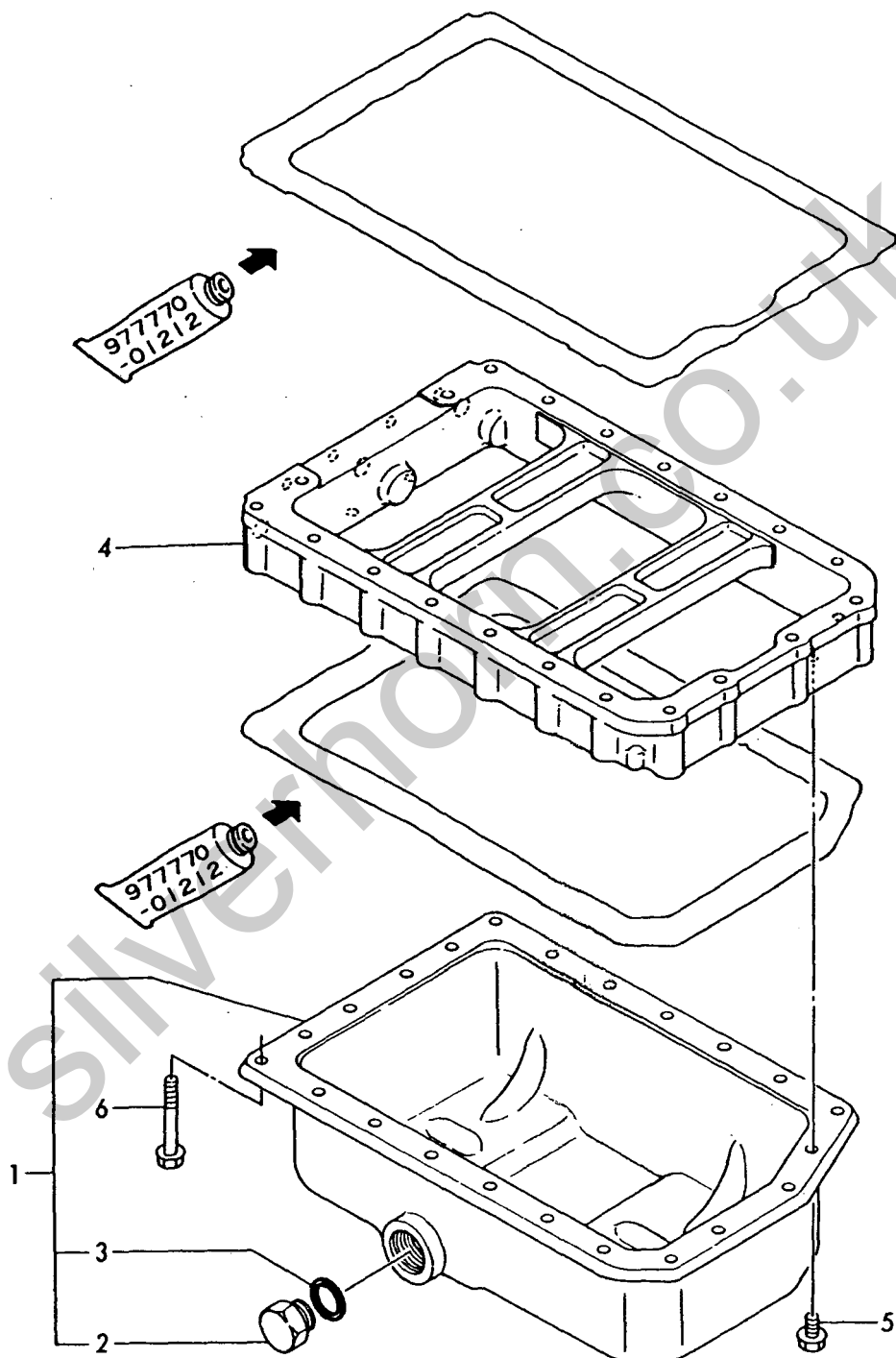
Fig. 6 オイルパン LUB. OIL SUMP
