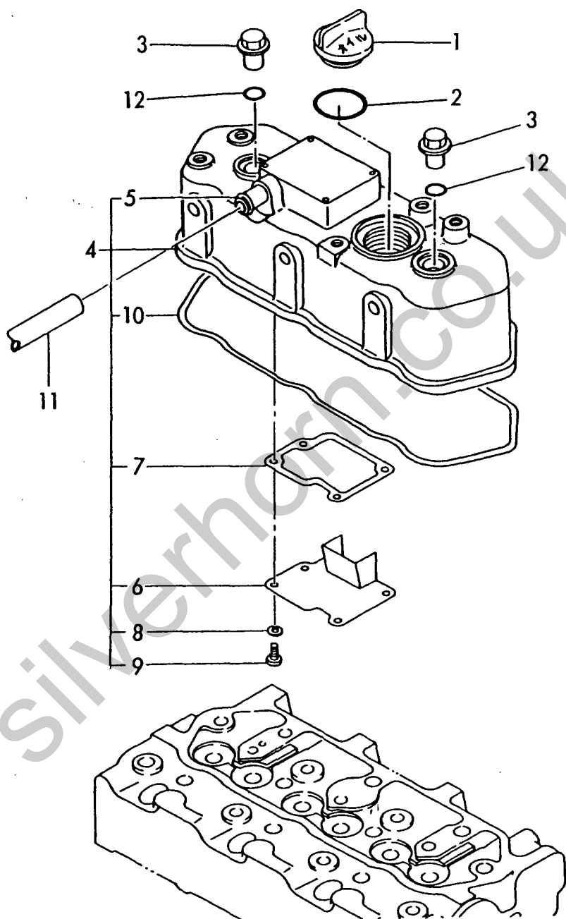
Fig. 9 ベンワンシツ BONNET
