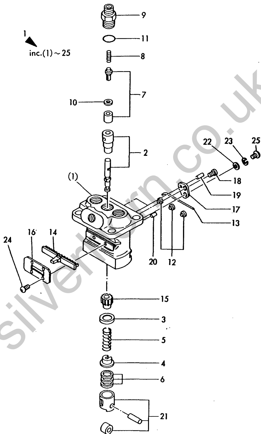
Fig. 23 FOフンシャポンプ FUEL INJECTION PUMP
